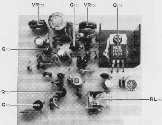
CONT UNIT(PB-1622)
