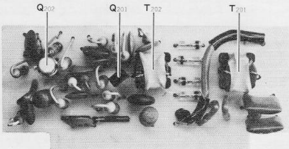
MIX UNIT(PB-1631)
